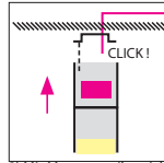
2) Mit Montageseil gesichertes Leuchtenprofil an Halteklammern einrasten.
